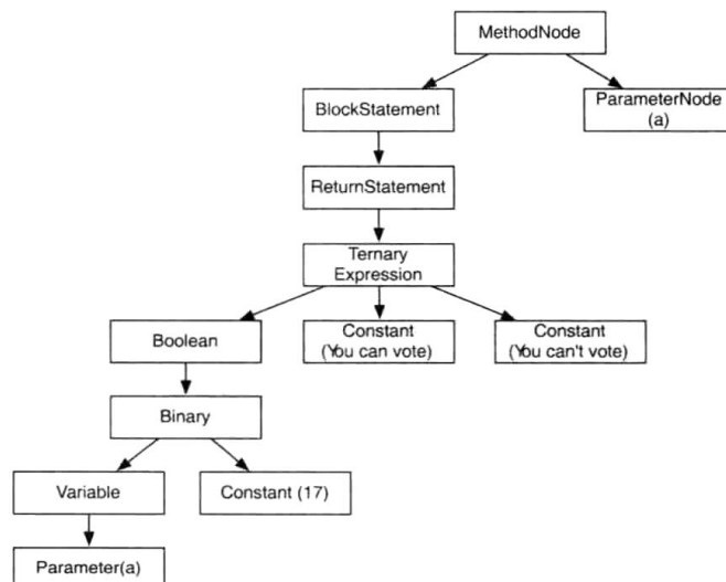
图16-1 canVote() 方法的AST
