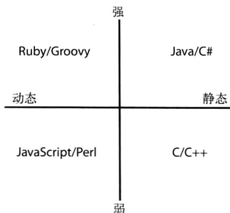
图3-1 所选语言的分类：静态对比动态、强类型对比弱类型
