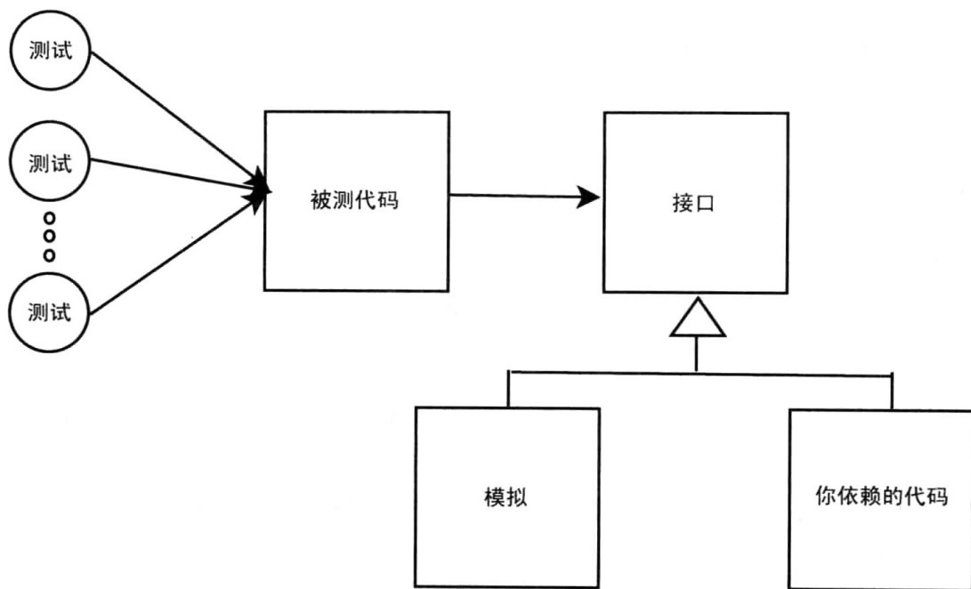
图18-1 单元测试中的模拟
