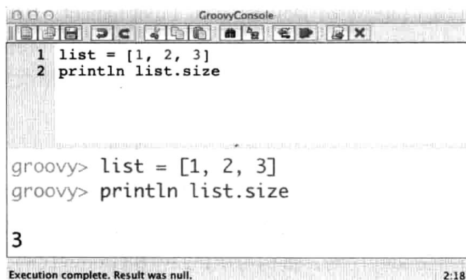
图1-1 使用groovyConsole
