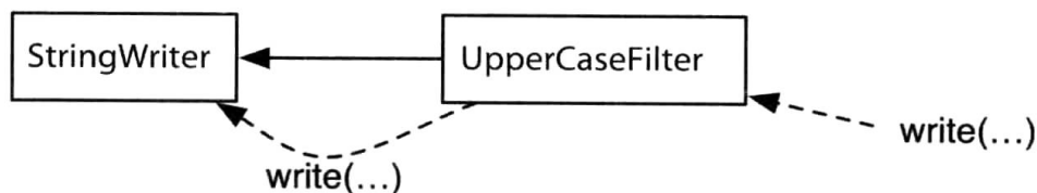
图13-1 将 UpperCaseFilter Mixin链接到一个 StringWriter 实例
