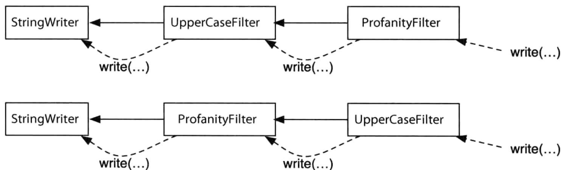
图13-2 将UpperCaseFilter和ProfanityFilter两个过滤器以不同顺序链接到一个StringWriter实例中
