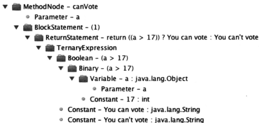
图16-2 在groovyConsole的AST浏览器视图中查看canVote()方法
