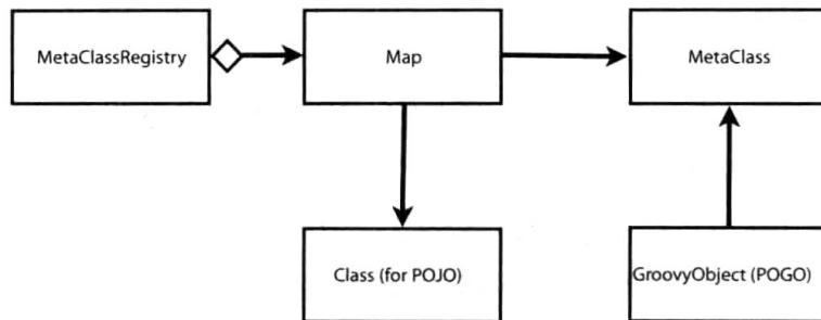
图11-1 POJO、POGO及其MetaClass
