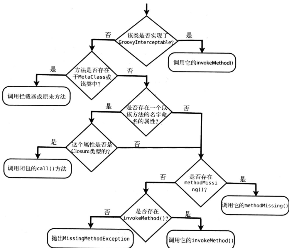
图11-2 Groovy如何处理POGO上的方法调用
