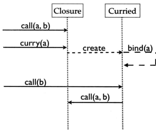
图4-2 对一个闭包进行科里化
