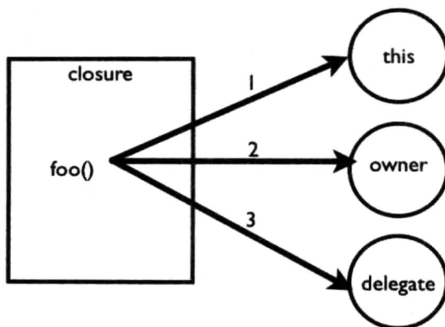
图4-3 闭包内的方法调用解析顺序
