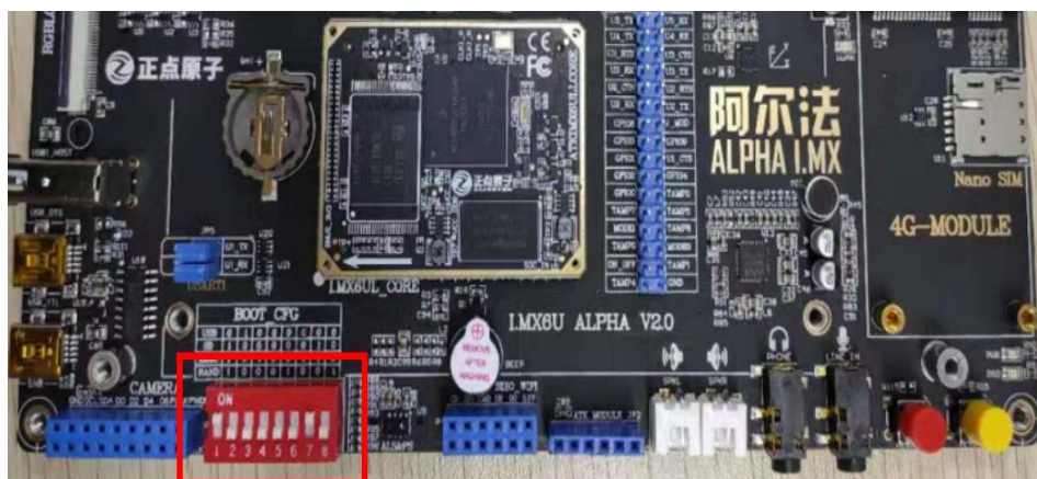
图 1.3.2-3 拨码开关 SD 卡启动
