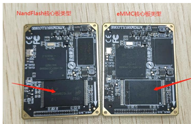
图 1.2.2-1 NandFlash 核心板和 EMMC 核心板
