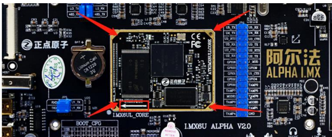
图 1.3.12-1 安装核心板
