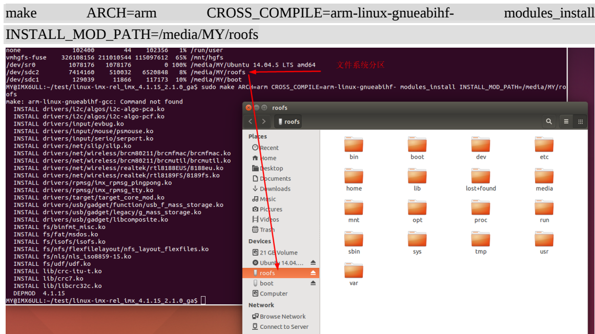
图 8.5.1-1 SD 卡加载模块
