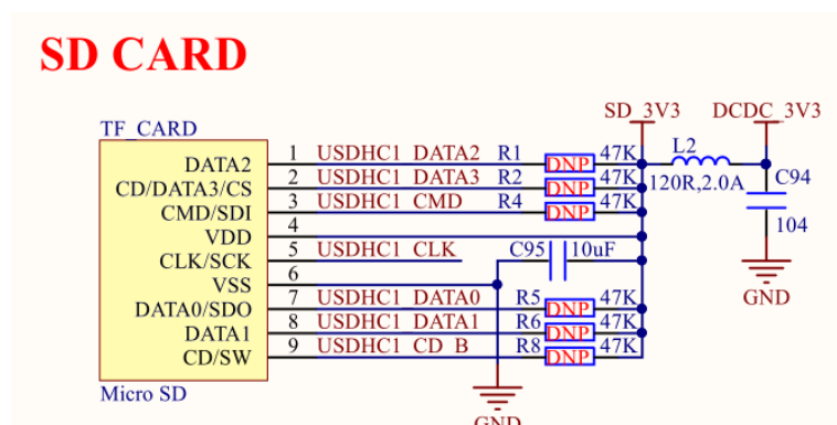
图 4.2.3-3 SD 卡接口原理图
