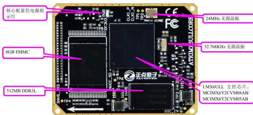
图 1.2.2-2 EMMC 核心板
