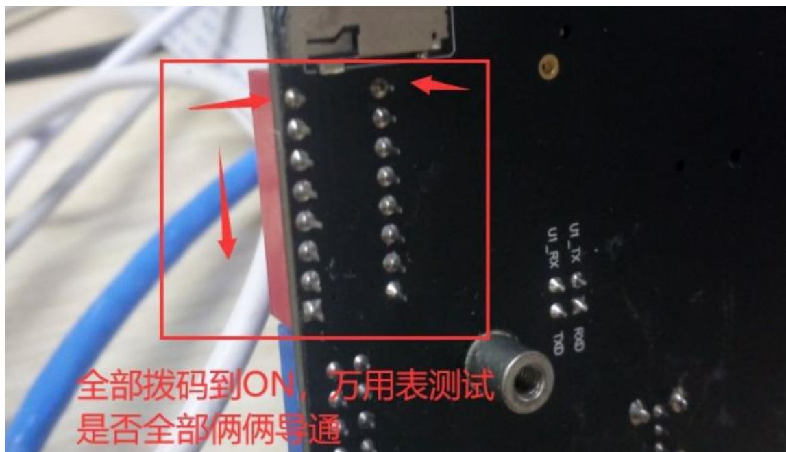
图 1.3.4-2 测量拨码开关导通性
