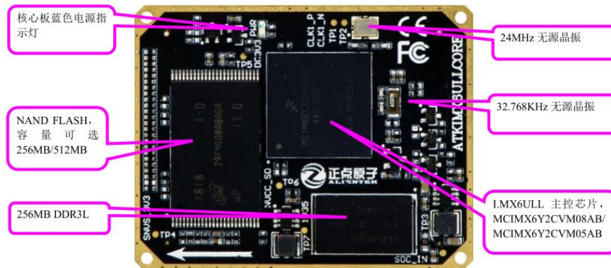
图 1.2.2-3 Nand Flash 核心板
