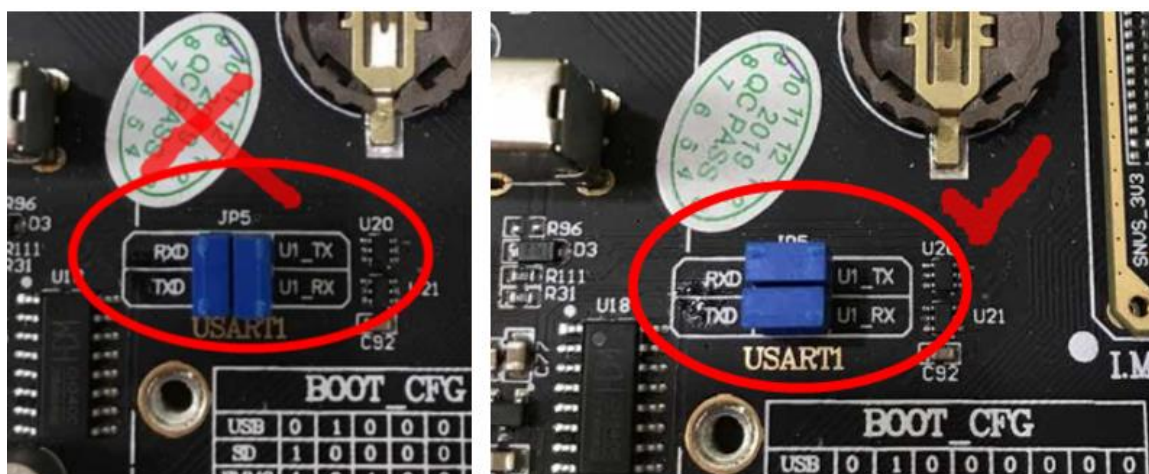
图 1.3.7-1 左图为错误示范, 右图为正确示范
