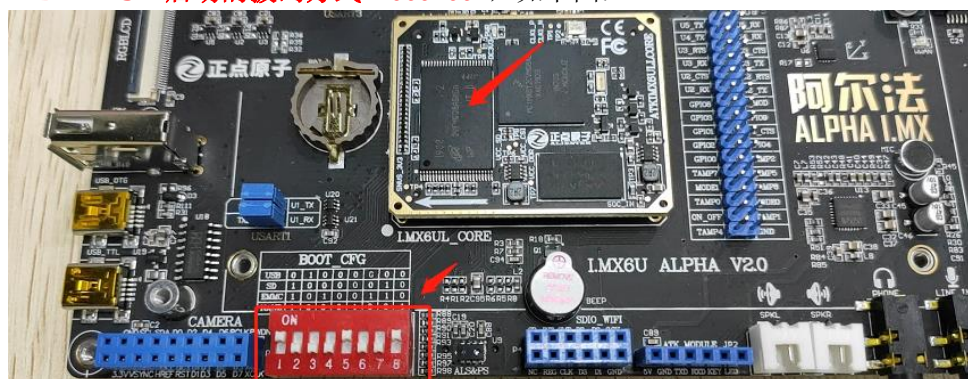
图 1.3.2-2 拨码开关 Nand Flash 启动
