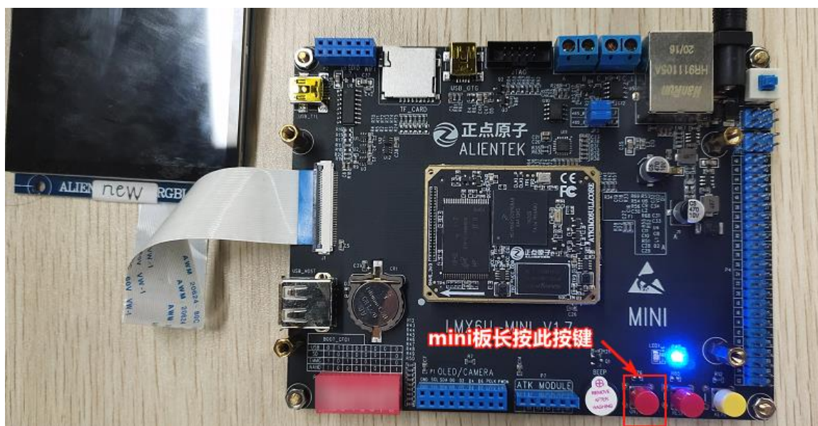
图 1.3.5-2 mini 板重启示意图
