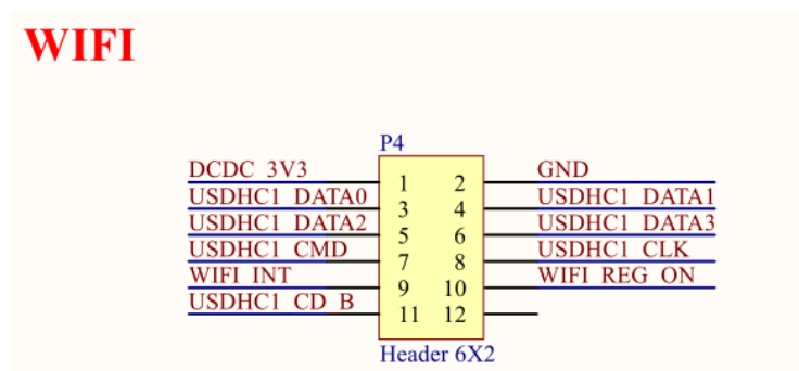
图 4.2.3-2 SDIO WIFI 接口原理图
