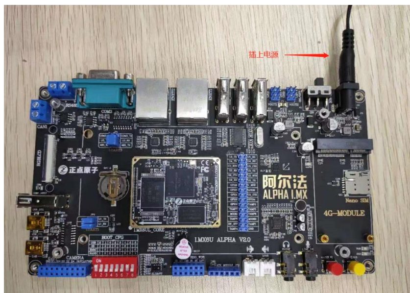
图 1.3.1-1 接入电源适配器
