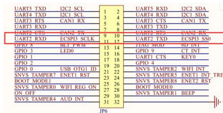
图 8.2.4-3 核心板原理图
