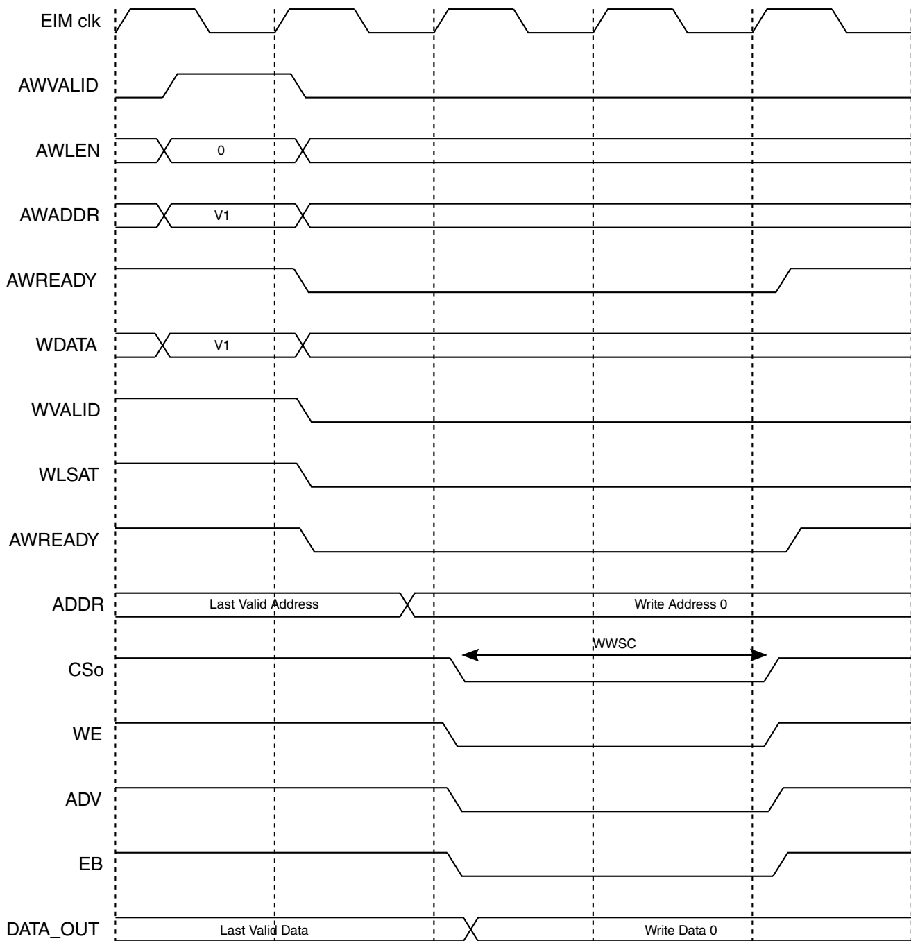
Figure 21-3. Write Access, WWSC=2, WCSA=0, WEA=0, WCSN=0, WEN=0, BEA=0, BEN=0, WAL=1
