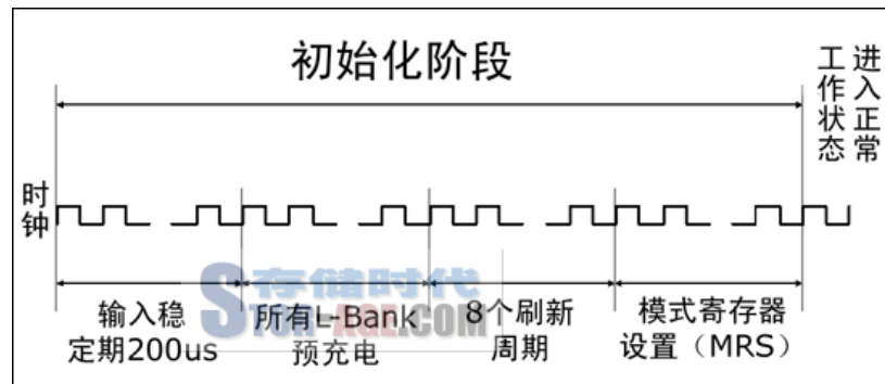
SDRAM 在开机时的初始化过程
