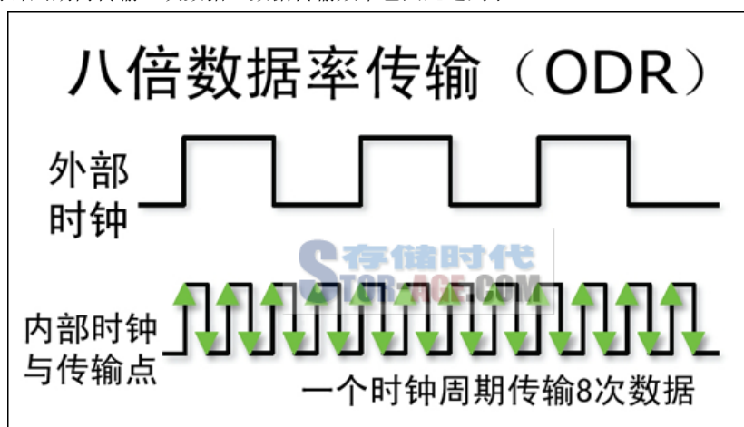
ODR 操作示意图
