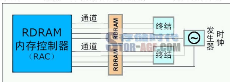
RDRAM 双通道结构
