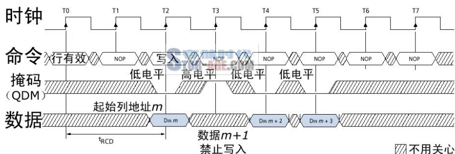
写入时数据掩码操作，DQM 立即生效，突发周期的第二笔数据被取消（上图可点击放大）
