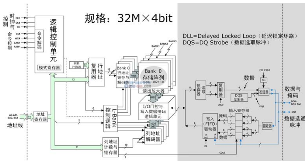
DDR 内存芯片的内部结构图，注意比较上文中 SDRAM 的结构图（上图可点击放大）
