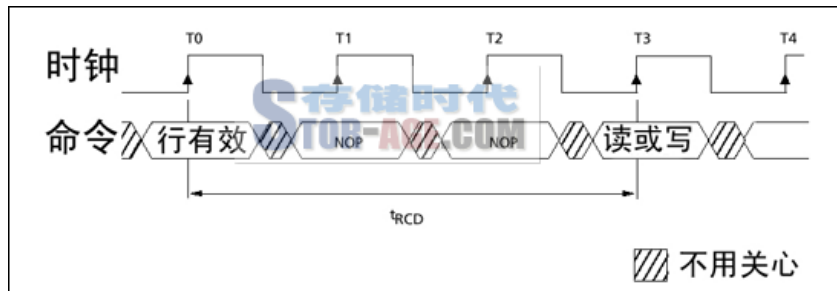
t_{RCD}=3 的时序图
