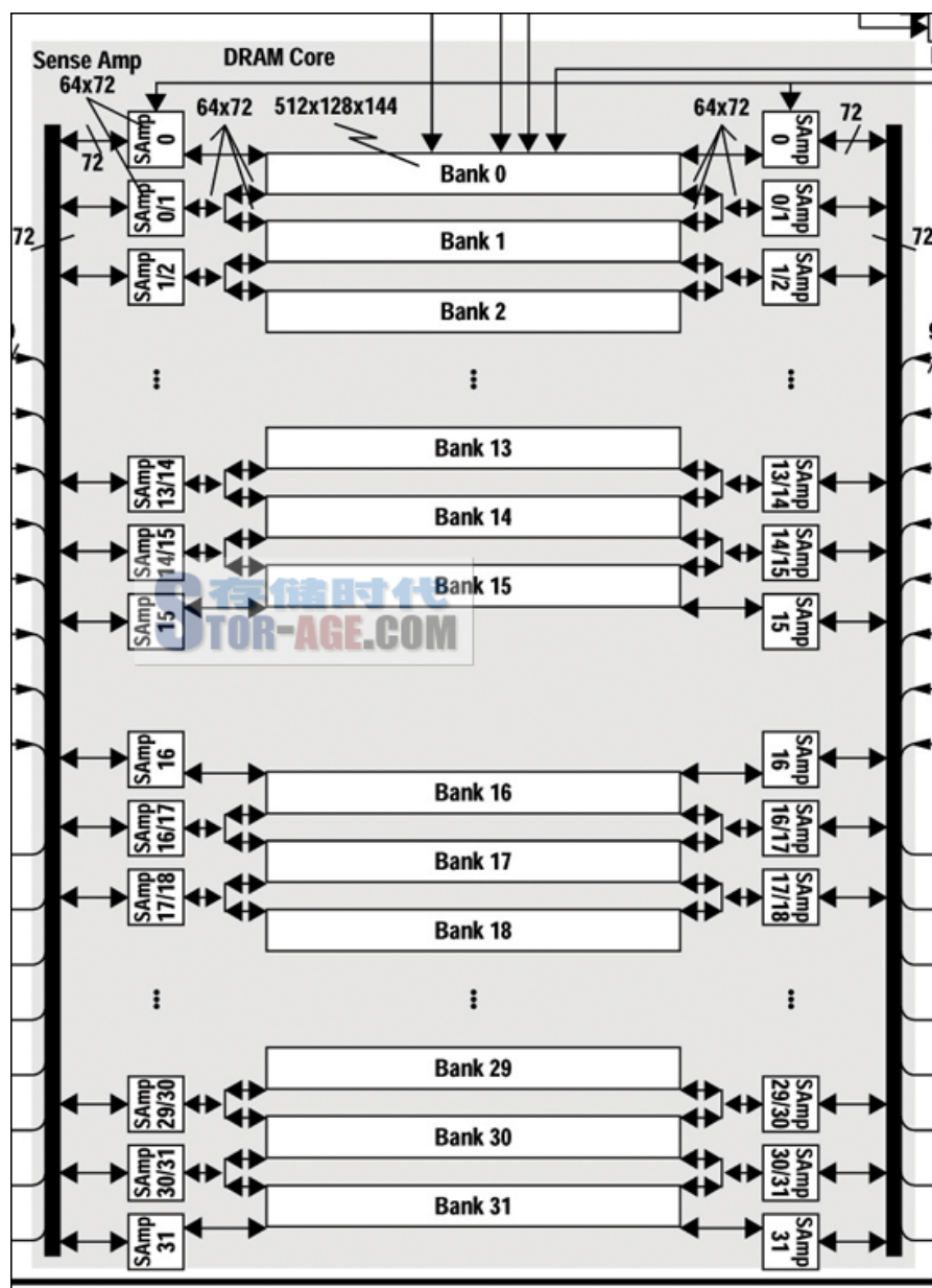
32s L-Bank 结构
