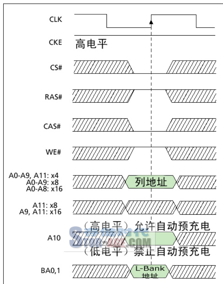
读写操作示意图，读取命令与列地址一块发出（当 WE# 为低电平即为写命令）
