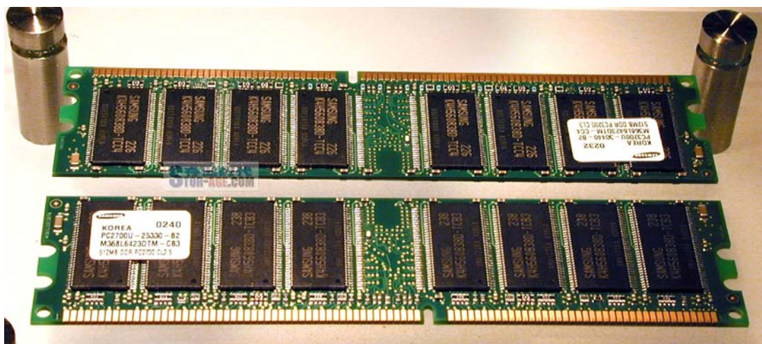
三星公司展示的 DDR-333（下）与 DDR-400（上）内存模组（点击放大）
