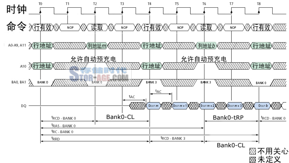
L-Bank 交错自动预充电/读取时序图（可点击放大）：L-Bank 0 与 L-Bank 3 实现了无间隔交错读取，避免了 tRP 对性能的影响 三、增加 PFHR 的方法
