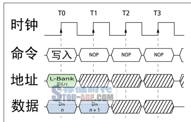
数据写入的时序图
