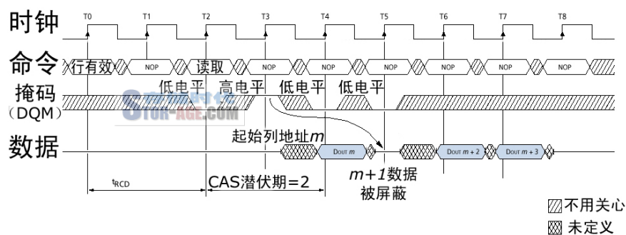
读取时数据掩码操作，DQM 在两个周期后生效，突发周期的第二笔数据被取消（上图可点击放大）
