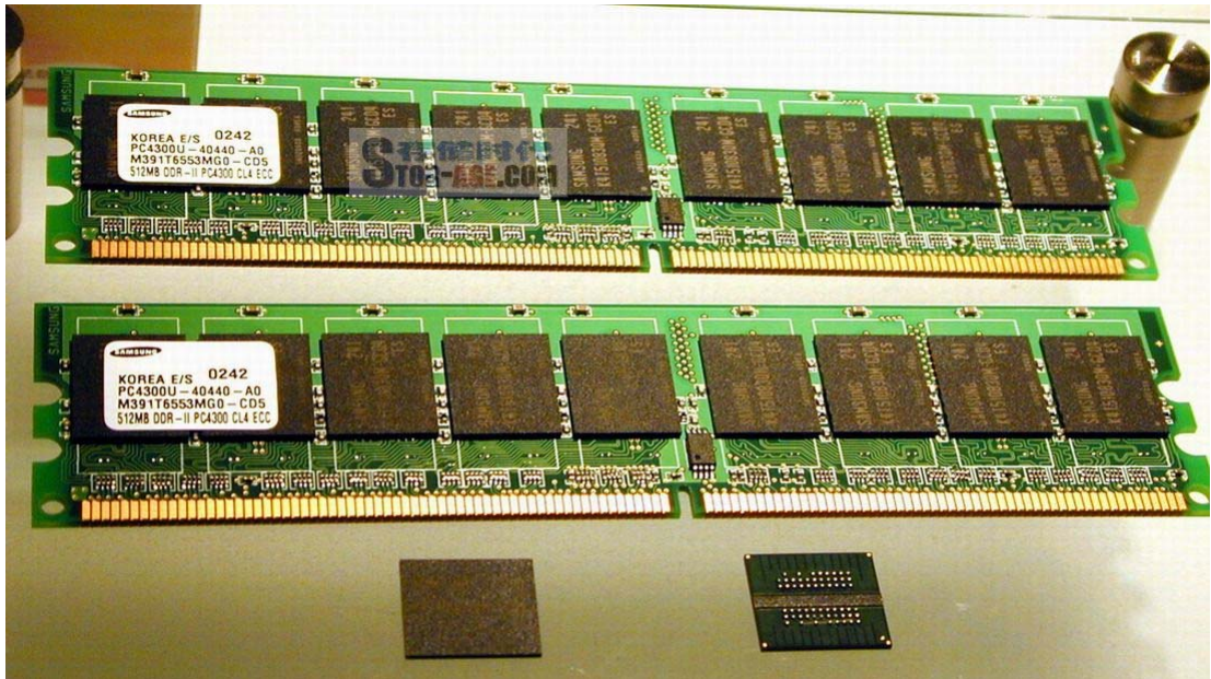
三星公司展示的 DDR-II 533 内存模组，模组标准为 PC4300，相应的，如果是 DDR-II 400 将是 PC3200
