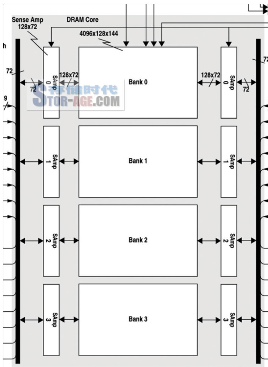
4i L-Bank 结构
