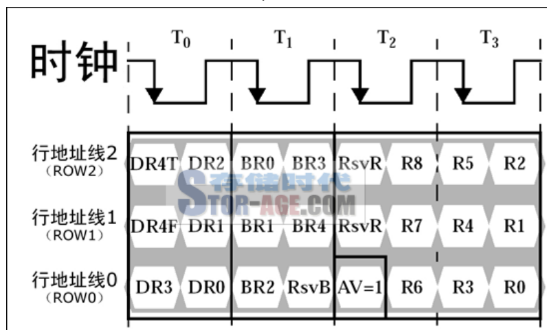
行读/写命令包的信息组成
