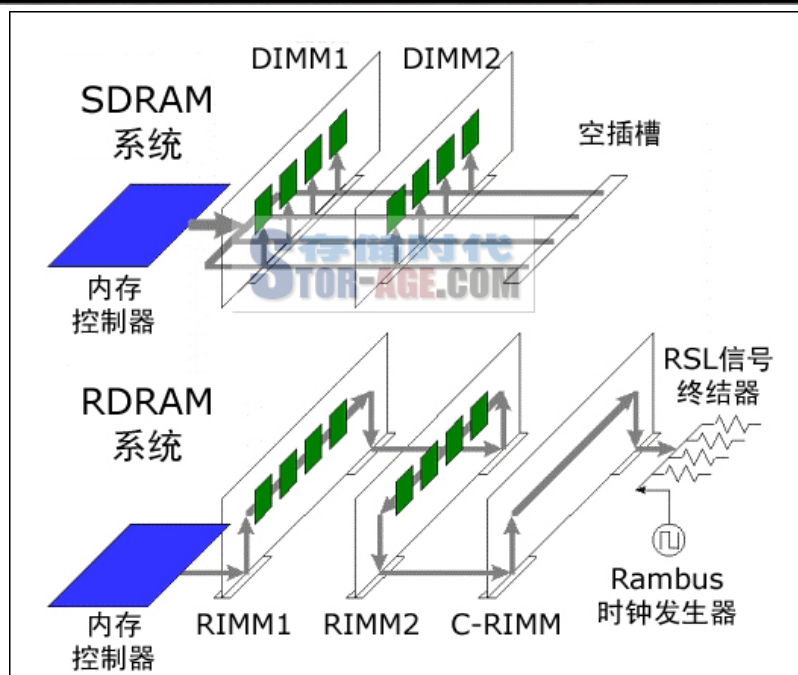
RDRAM 与传统 SDRAM 的架构比较
