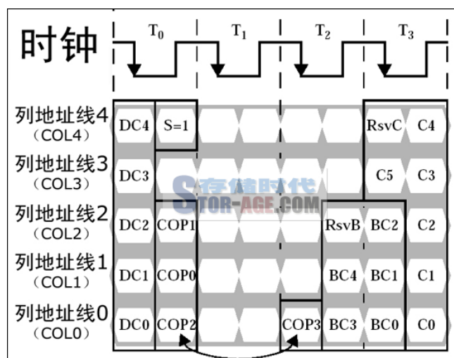
列读/写命令包的信息组成
