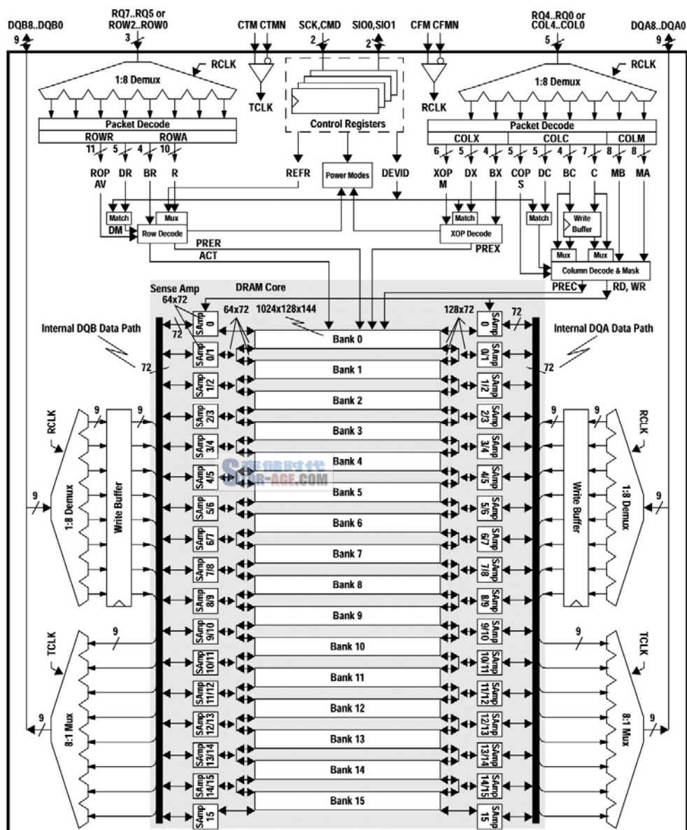
16d L-Bank 结构（上图可点击放大）
