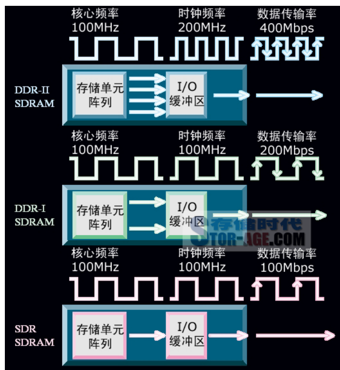
DDR-II、DDR 与 SDRAM 的操作时钟比较
