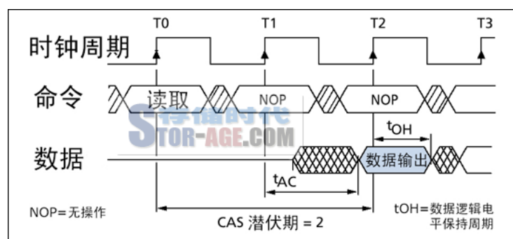
CL=2 与 tAC 示意图
